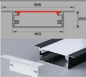
(EMB40X20) 2M PERFIL EMBUTIR PRETO/BRANCO CX-100
