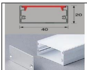
(SOB40X20) 2M PERFIL SOBREPOR PRETO/BRANCO CX-120
