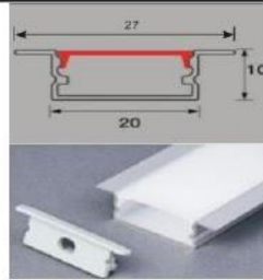
(EMB20X10) 2M PERFIL EMBUTIR PRETO/BRANCO CX-120
