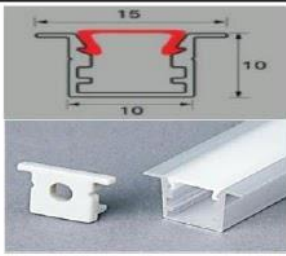
(EMB10X10) 2M PERFIL EMBUTIR PRETO/BRANCO CX-120
