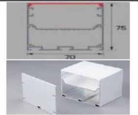
PERFIL 7075 PRETO/BRANCO
