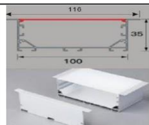
(EMB100X35) PERFIL EMBUTIR PRETO / BRANCO
