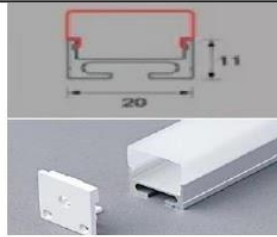
PERFIL 045 PRETO/BRANCO
