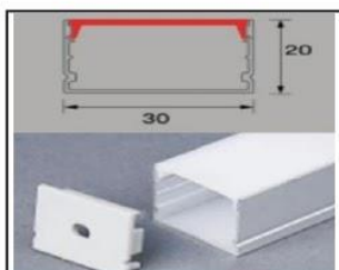
(SOB30X20) 2M PERFIL SOBREPOR PRETO CX-120
