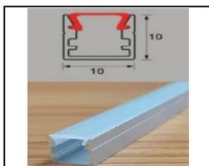
(SOB10X10) 2M PERFIL SOBREPOR PRETO/BRANCO CX-120
