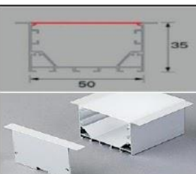
(EMB50X35) 2M PERFIL EMBUTIR PRETO/BRANCO CX-
