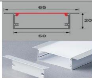
(EMB50X20) 2M PERFIL EMBUTIR PRETO/BRANCO CX-120
