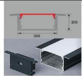
(EMB30X20) 2M PERFIL EMBUTIR PRETO/BRANCO CX-120
