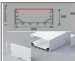
(SOB50X35) 2M PERFIL SOBREPOR PRETO/BRANCO CX-
