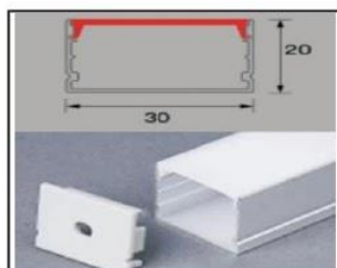
(SOB30X20) 1M PERFIL SOBREPOR BRANCO CX-120
